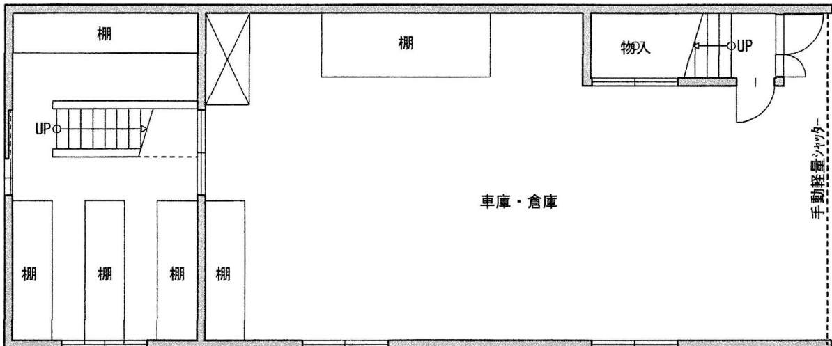
1階平面図 S=1/100 (29.7坪)
