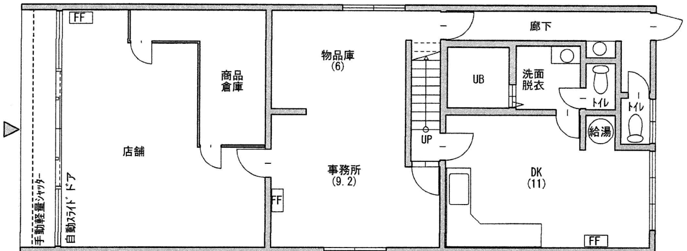
1階平面図 S=1/100 (29.7坪)
