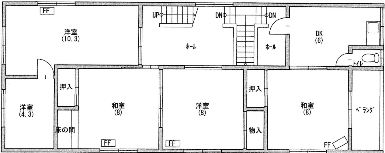
2階平面図 S=1/100 (30.0坪)
