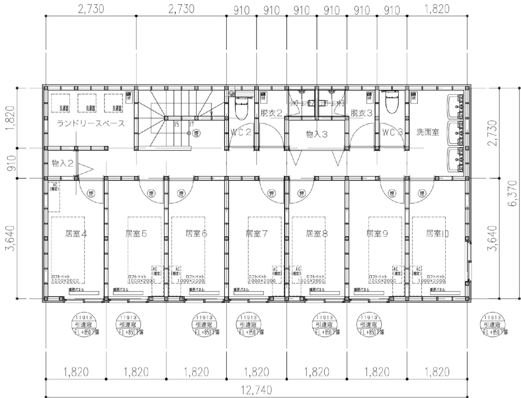
2階平面図
