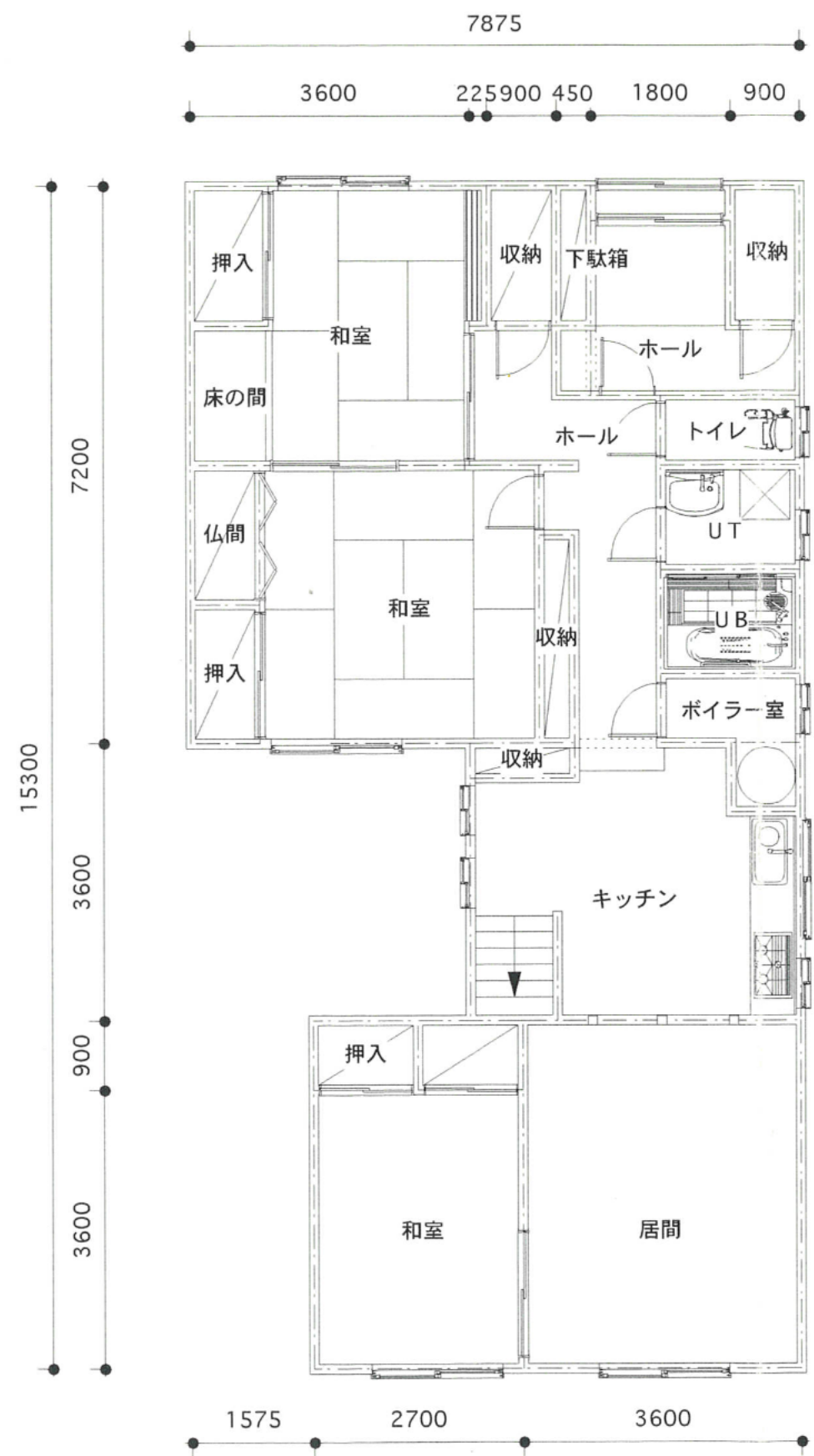
1F部分
